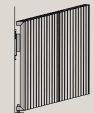
Sezione Boiserie Cannettata / Section of Channeled Wall Panels
